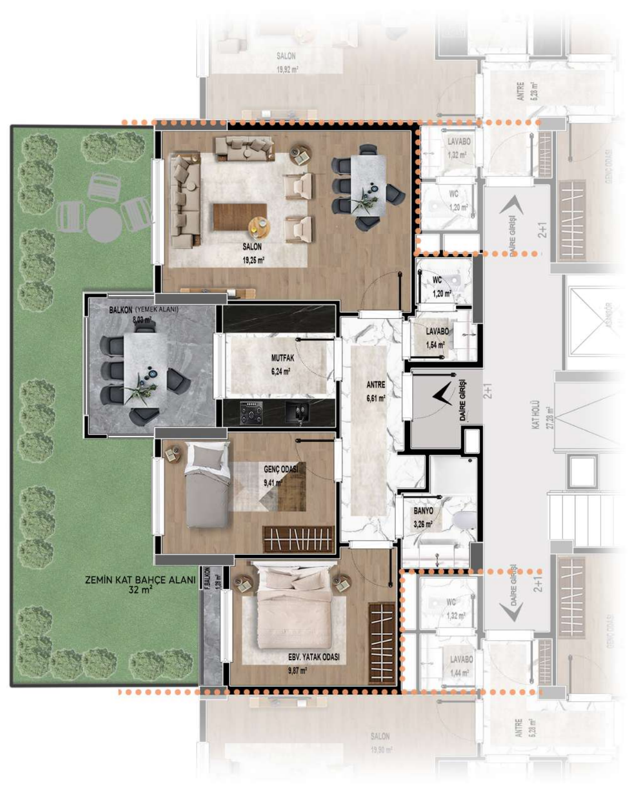
A-C BLOK ZEMİN KAT ORTA DAİRE PLANI
